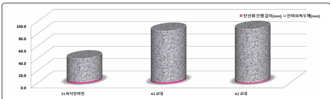
[그림 7.3.6] 탄산화깊이 및 잔여피복두께 측정결과
