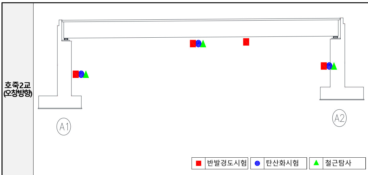
[그림 7.3.2] 비파괴시험 위치도
