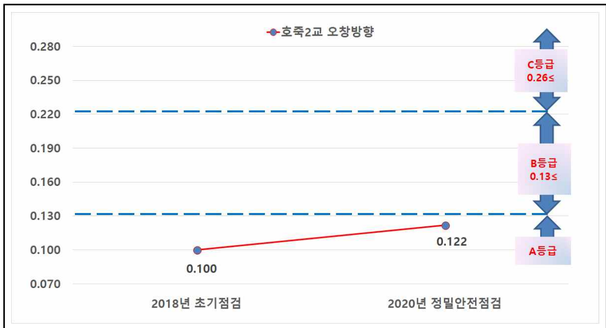
[그림 7.4.1] 호죽2교 오창방향 상태평가 결과 비교 그래프
